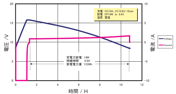
負荷出力カーブ
