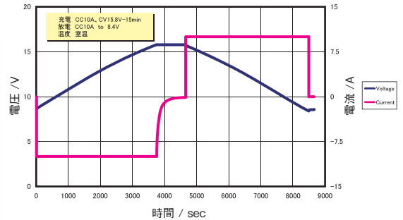
負荷出力カーブ
