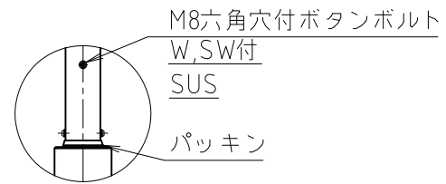
A部詳細図 (S=1/10)
