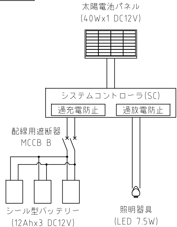
配線図
